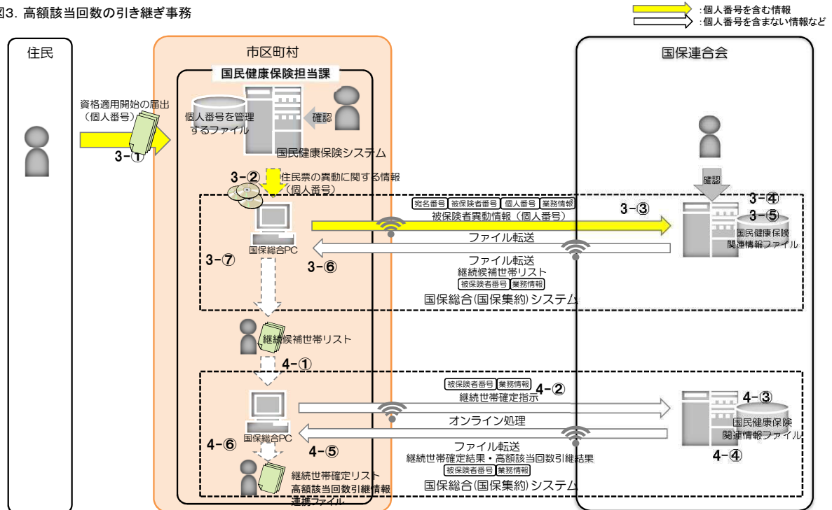
図3. 高額該当回数の引き継ぎ事務
