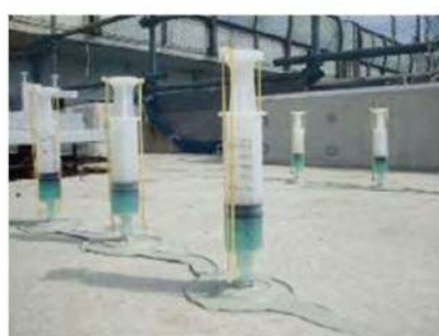
従来技術（低圧注入工法）
