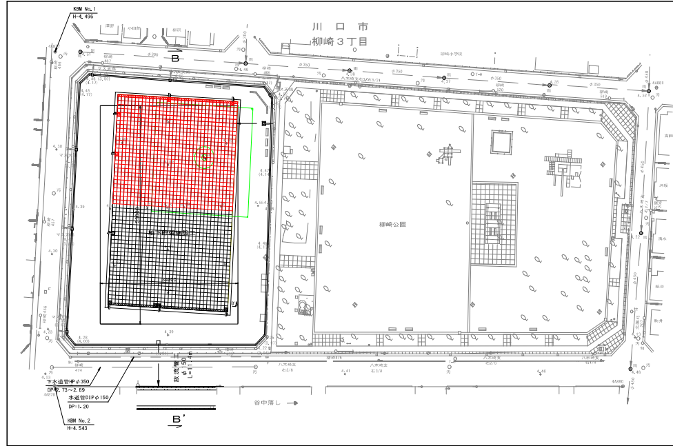
プラスチック貯留施設出来形確認
