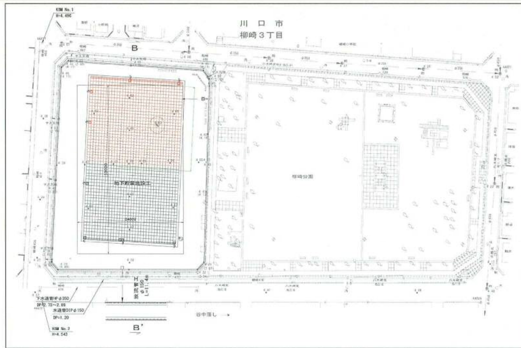
プラスチック貯留施設出来形確認
