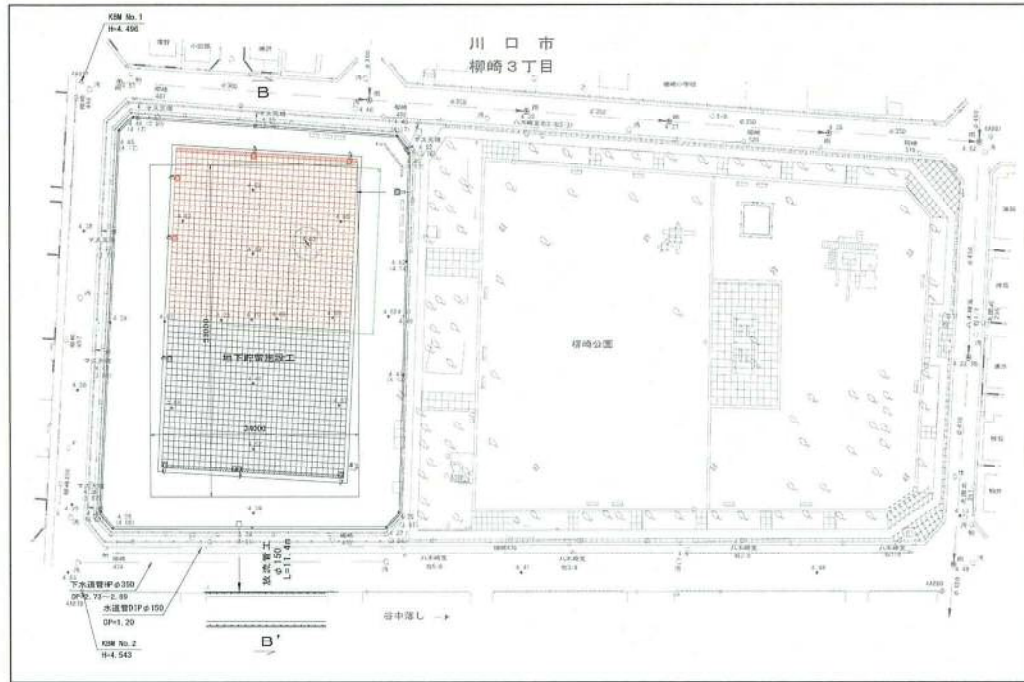
流入管接続状況
