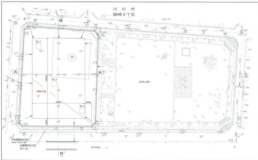
防球ネット復旧状況
