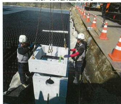
流入柵設置状況
