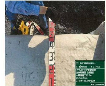
プラスチック貯留施設出来形確認
