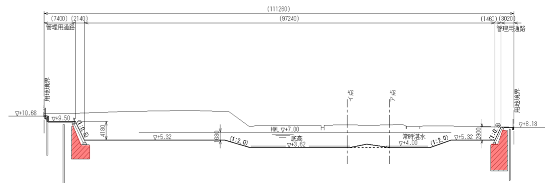
B-B 断面図
