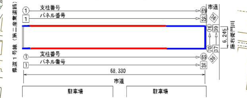
全体平面図
