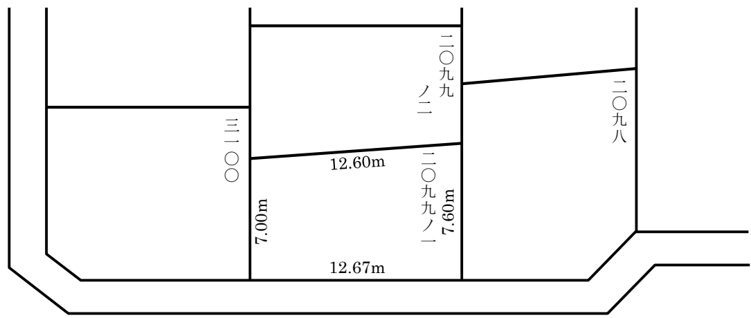
境 界 表 示 図
