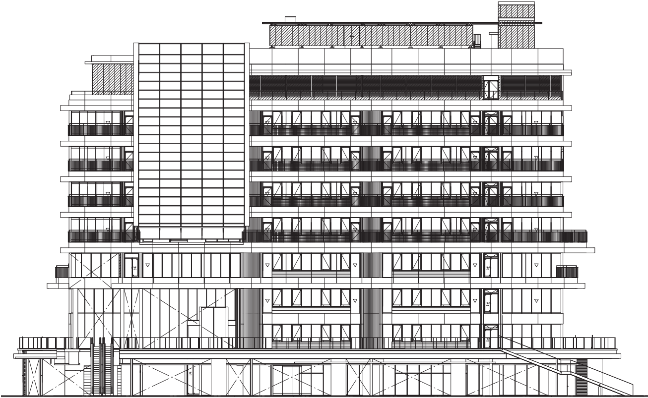
北側立面図
