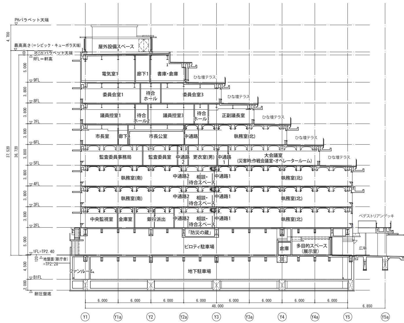
断面図 (X2-X3間)
