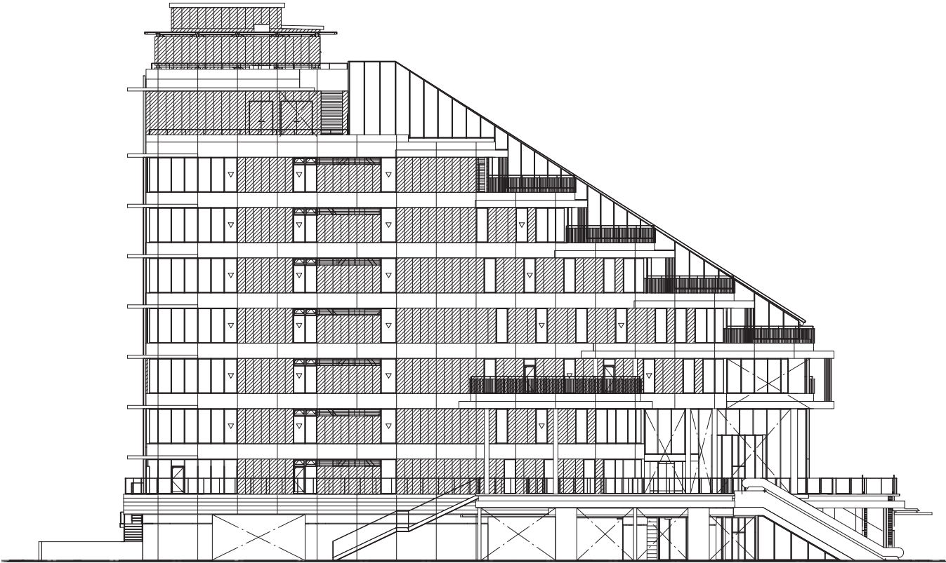
東側立面図
