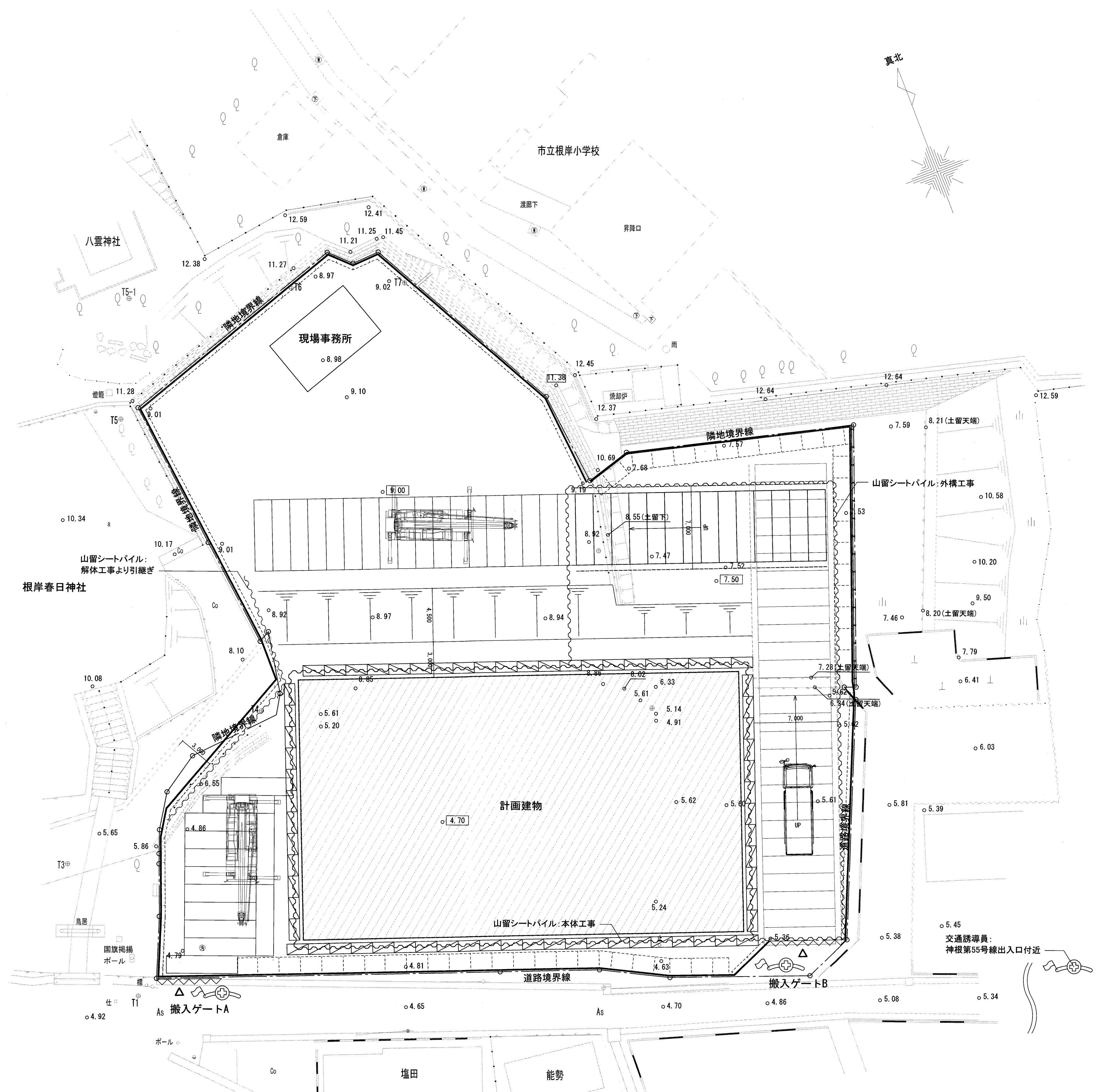
配置図 S=1/200 (A1)
