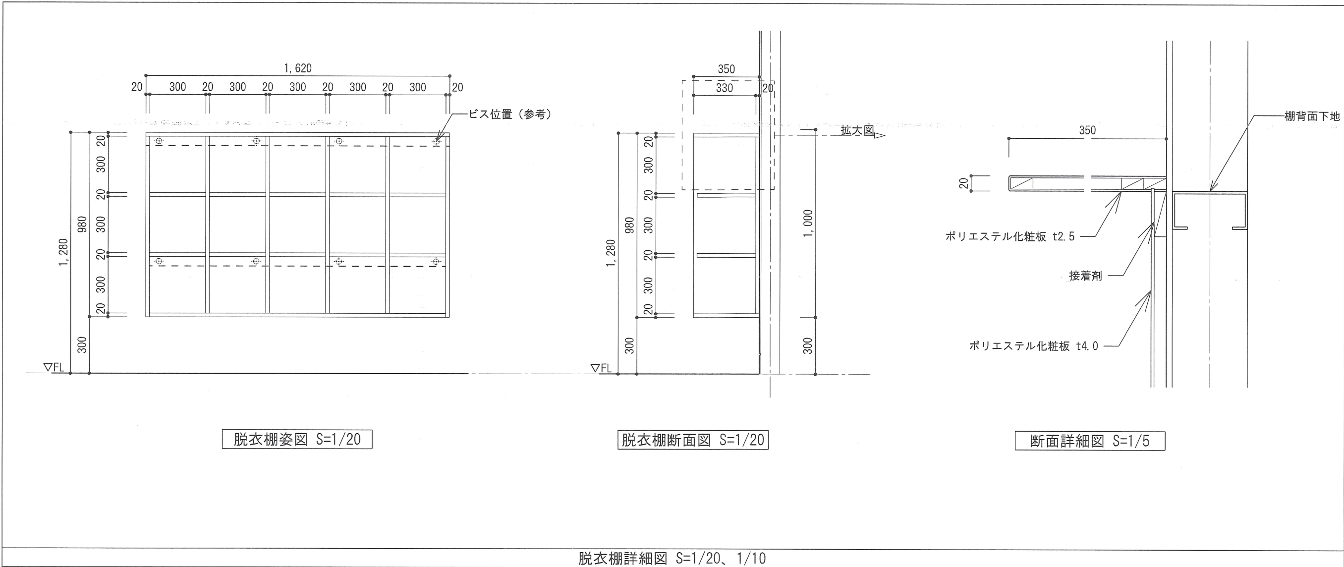
脱衣棚詳細図 S=1/20、1/10
