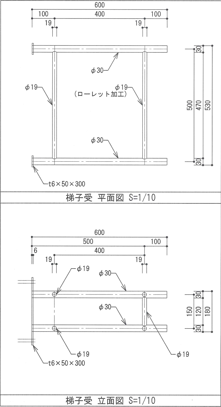
梯子受 立面図 S=1/10
