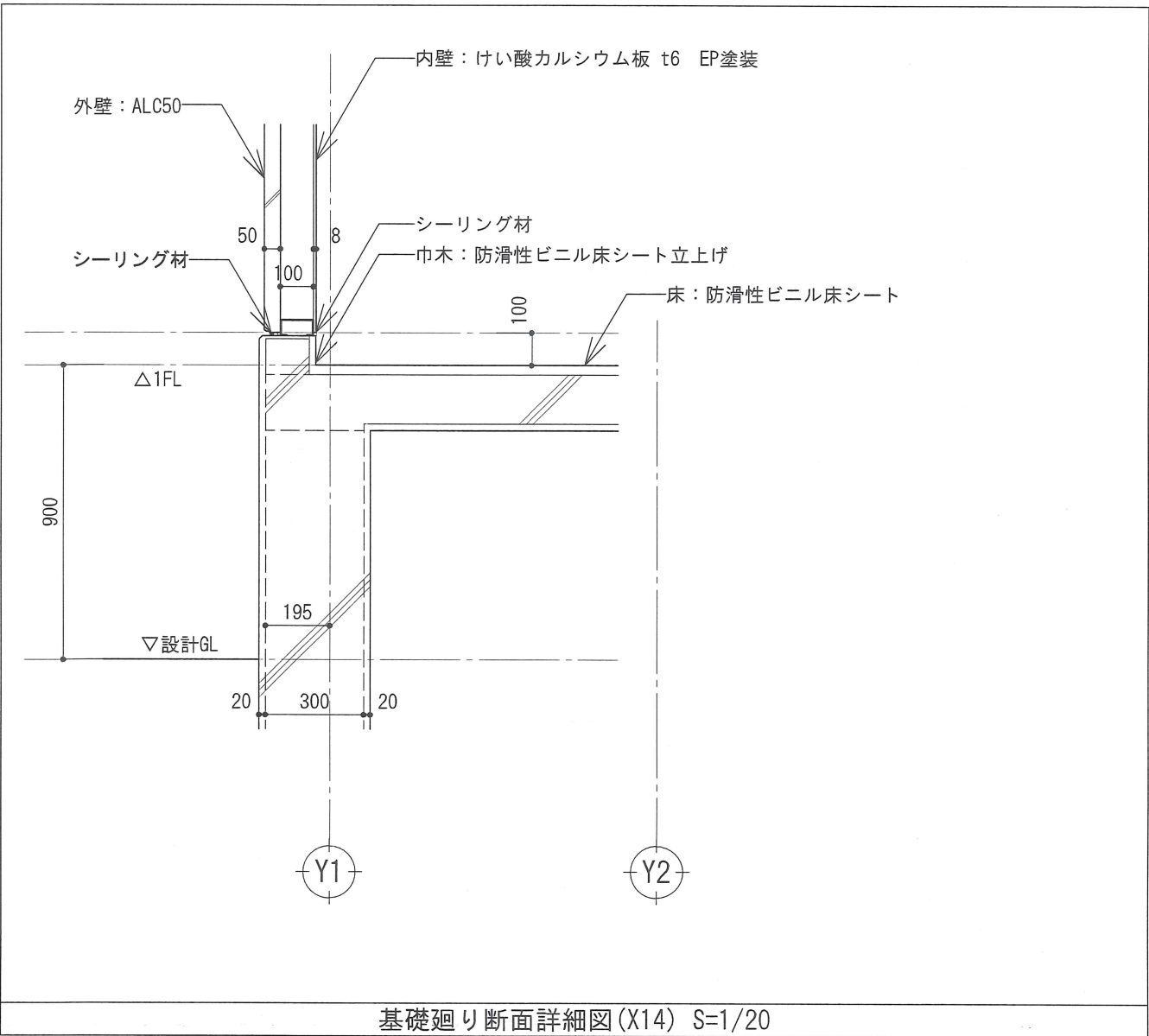
基礎廻り断面詳細図(X14) S=1/20
