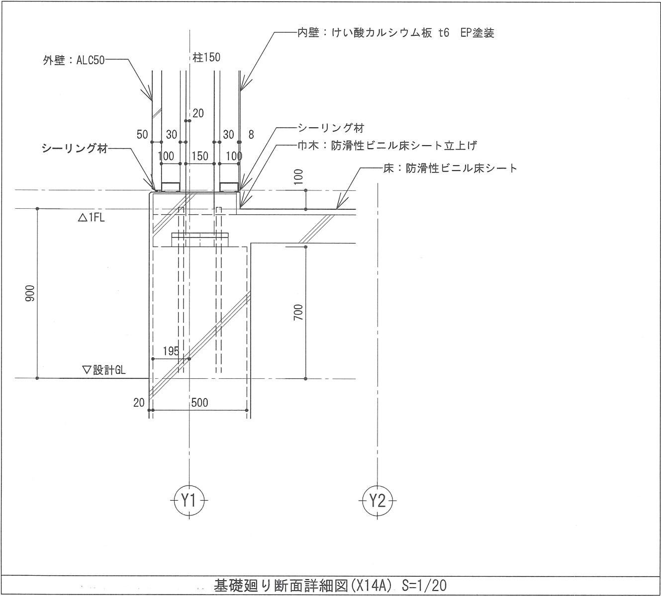
基礎廻り断面詳細図(X14A) S=1/20
