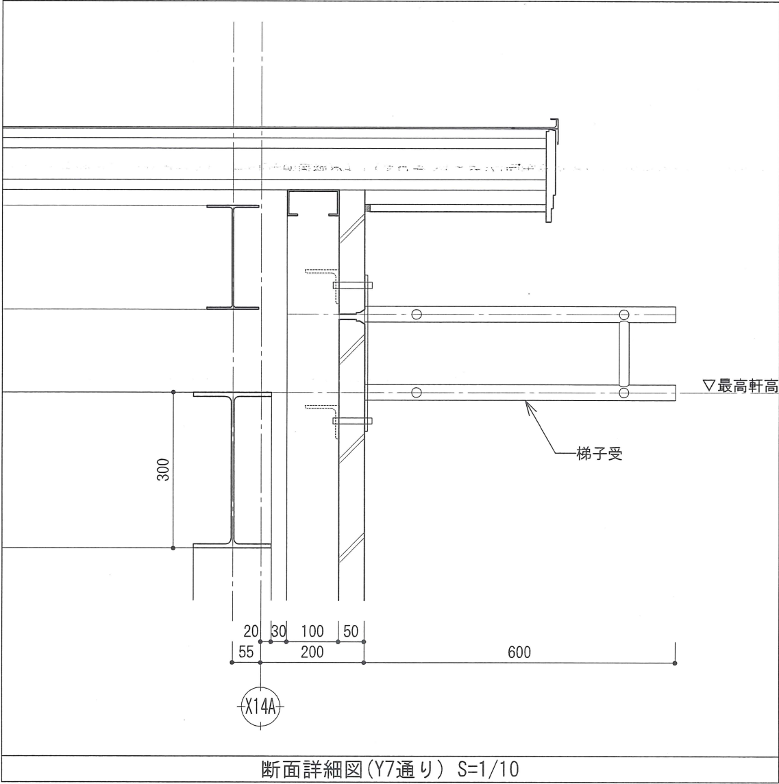
断面詳細図(Y7通り) S=1/10
