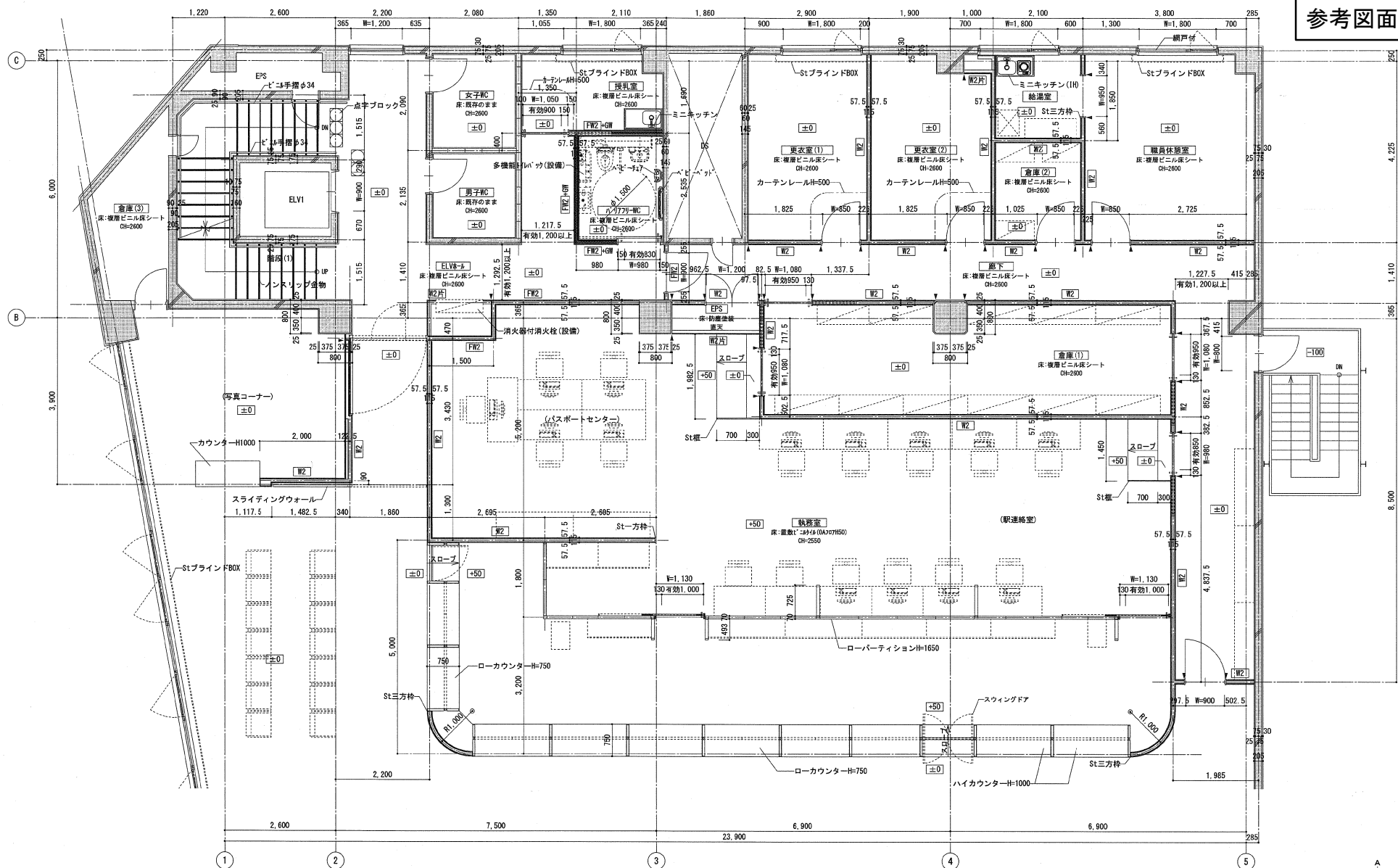
3階平面詳細図 S=1/60
