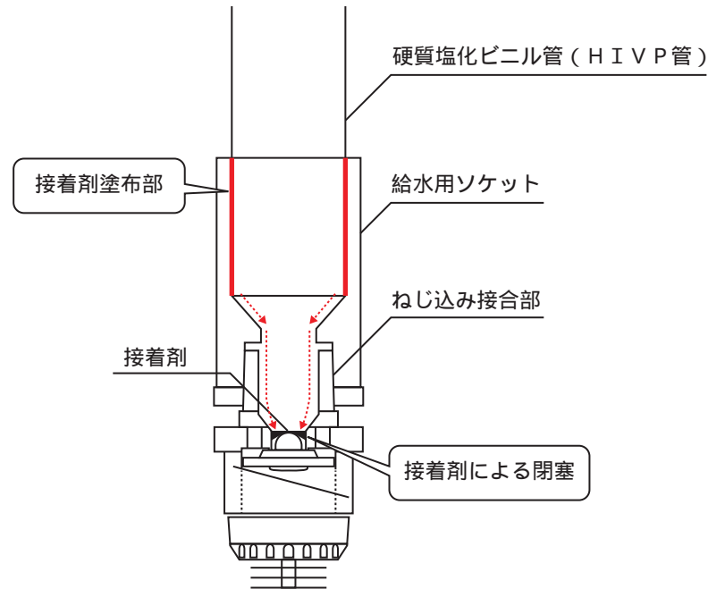
接着剤塗布部からスプリンクラーヘッド部分に流下する接着剤(推定)
