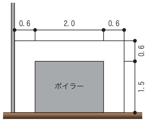
(立面図)
