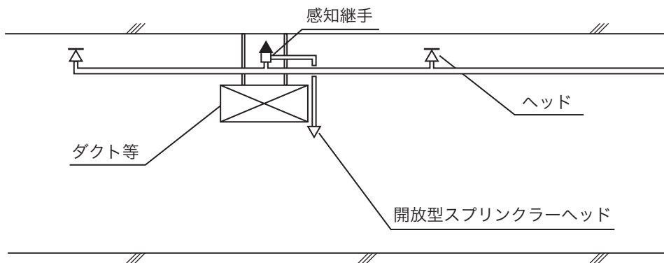
（感知継手を設ける場合の例）
