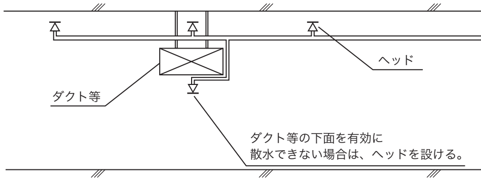
（感知継手を設けない場合の例） 第3－21図
