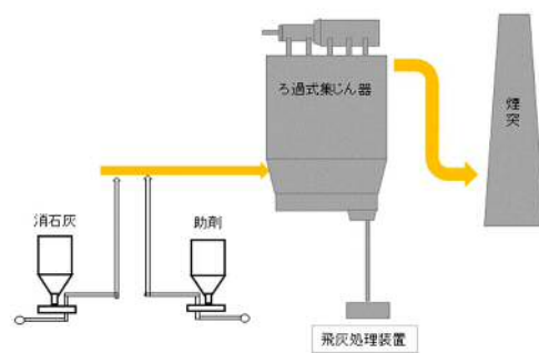
巻末図4-3 乾式法のフロー例
