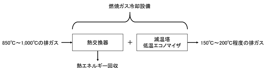
図 3-5-1 余熱の回収方法
