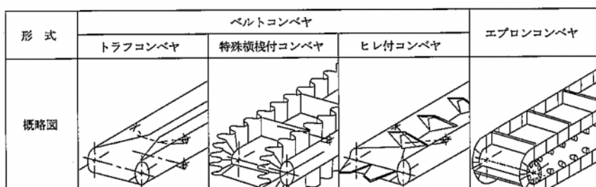
巻末図 5-1 搬送コンベヤの例
