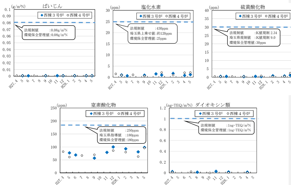
巻末図3-1 戸塚環境センター排ガス処理に関する維持管理の状況
