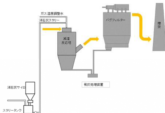
巻末図4-4 半乾式法のフロー例
