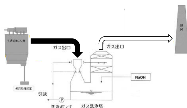
巻末図4-5 湿式法のフロー例
