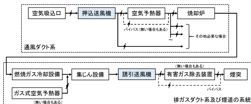
巻末図4-8 通風設備のフロー例
