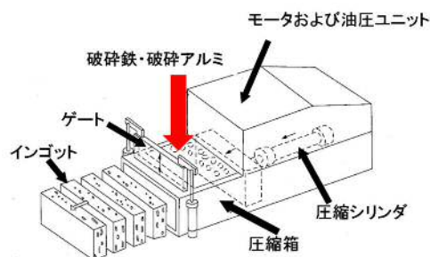
巻末図5-2 再生設備の例
