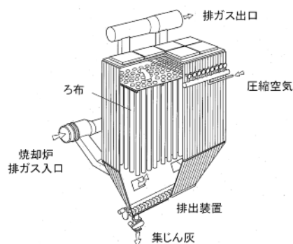
巻末図4-2 バグフィルタの構造
