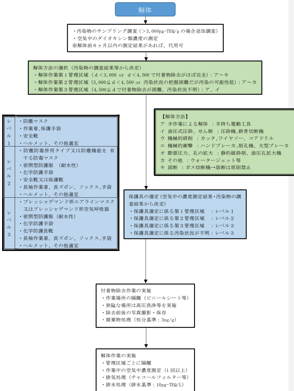
図3-7-1 焼却炉解体工事調査・対策フロー
