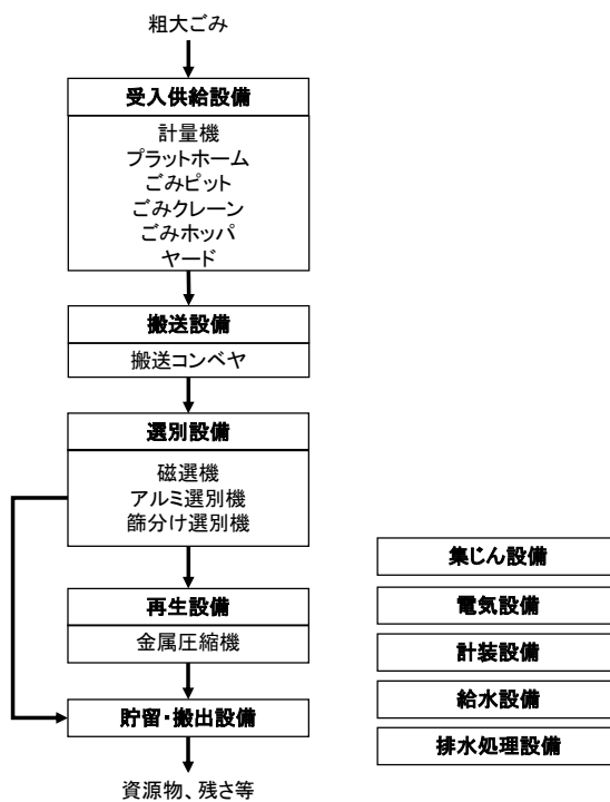
図 3-6-2 新粗大ごみ処理施設主要設備のブロックフロー（例）
