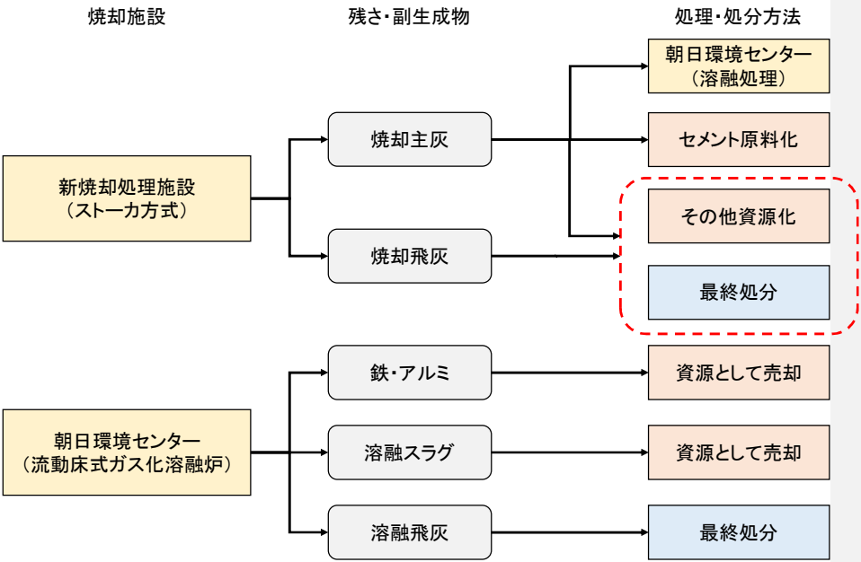
図3-4-1 焼却残さの処理フロー
