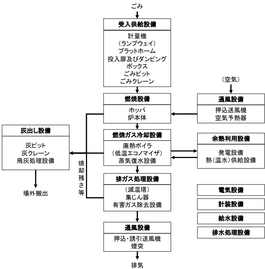
図3-6-1 主要設備のブロックフロー（例）
