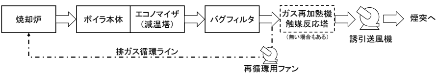
卷末図 4-9 排ガス循環システムのフロー例
