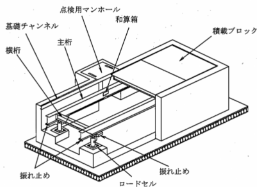
巻末図4-1 ロードセル方式のイメージ図
