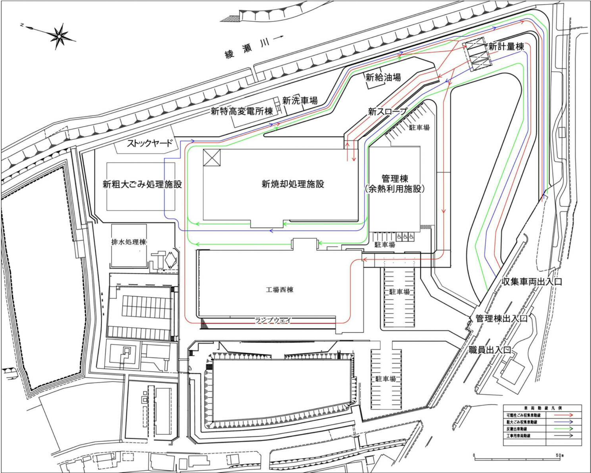
図3-6-3① 配置計画 (案1)
