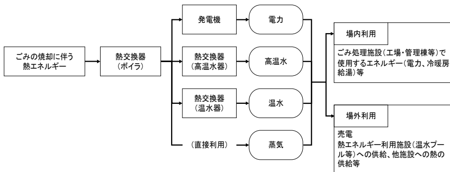
図 3-5-2 熱エネルギーの利用方法例
