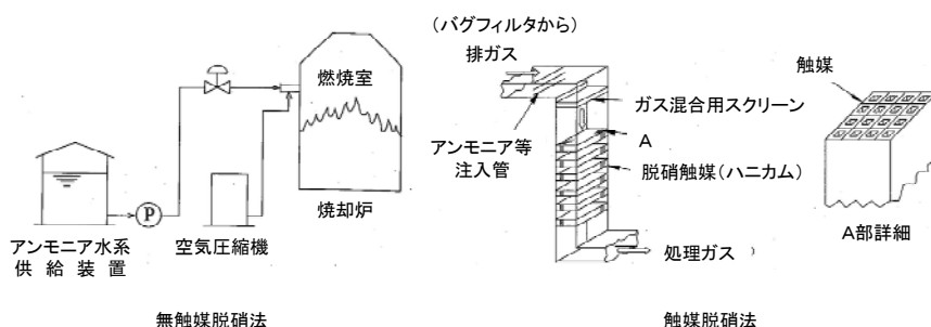
巻末図 4-6 無触媒脱硝法と触媒脱硝法の概略図
