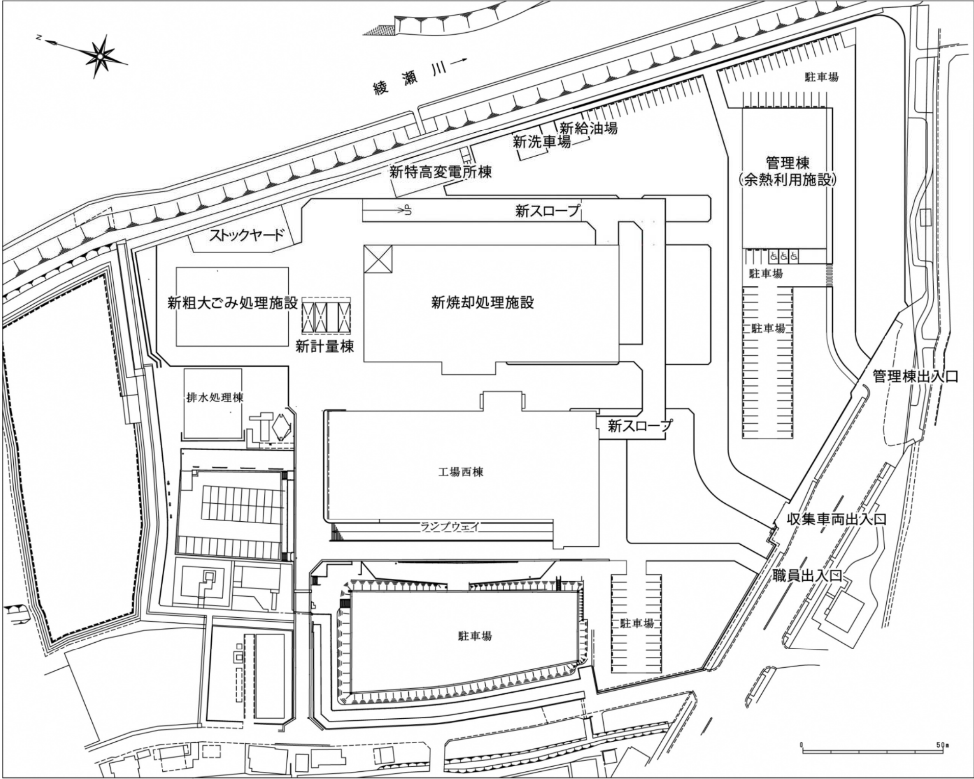
図3-6-3② 配置計画（案2）
