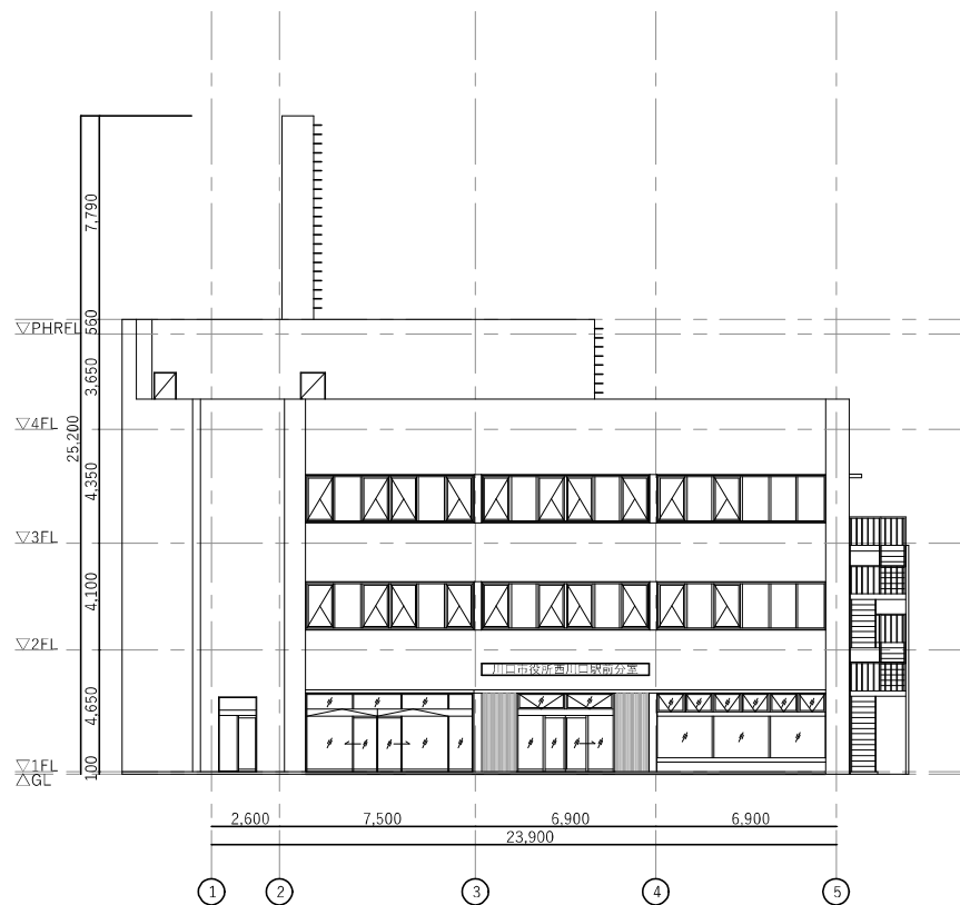
南立面图
