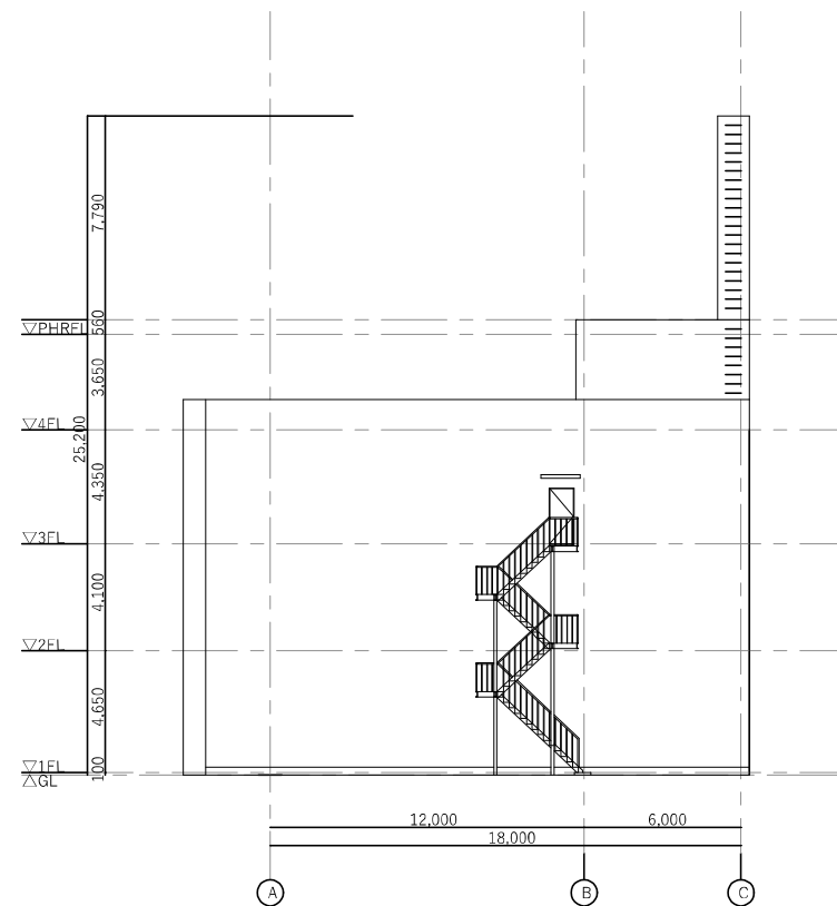
東立面图
