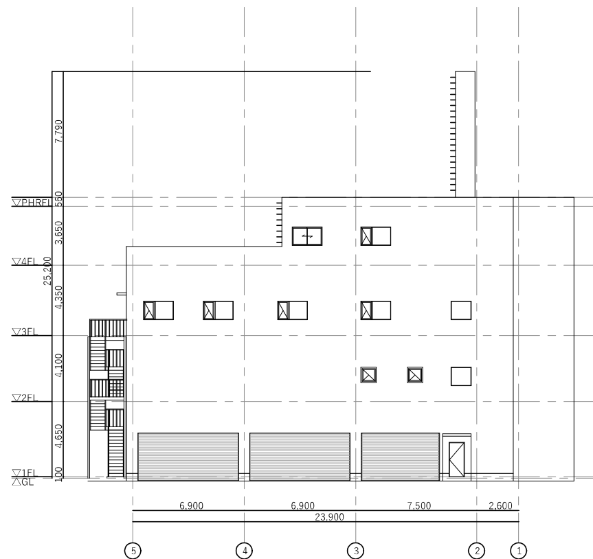
北立面图
