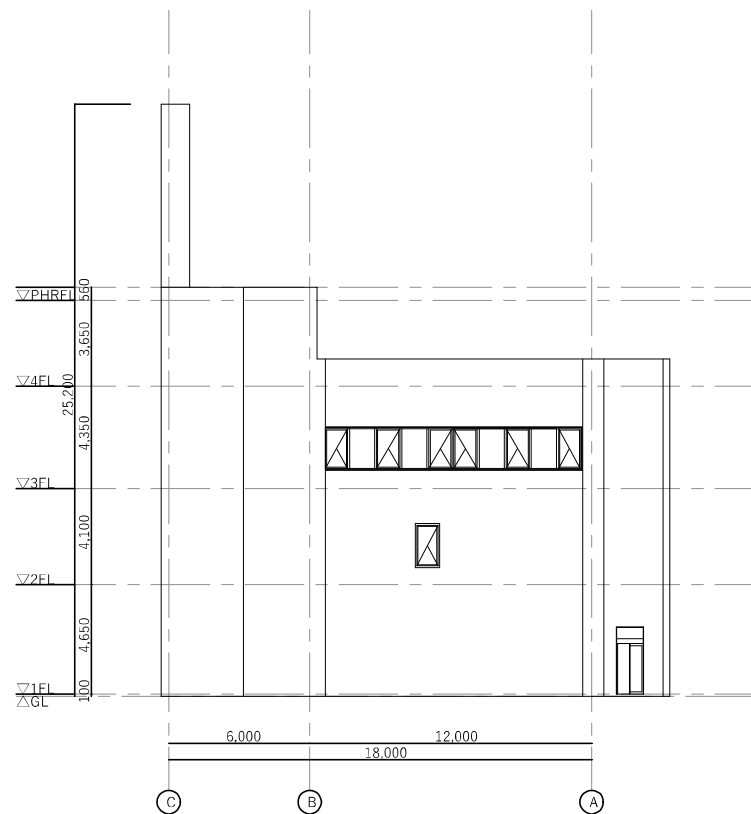
西立面图
