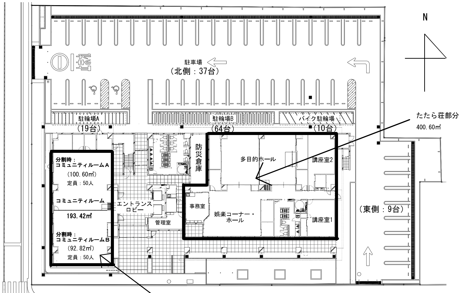
1階平面図
