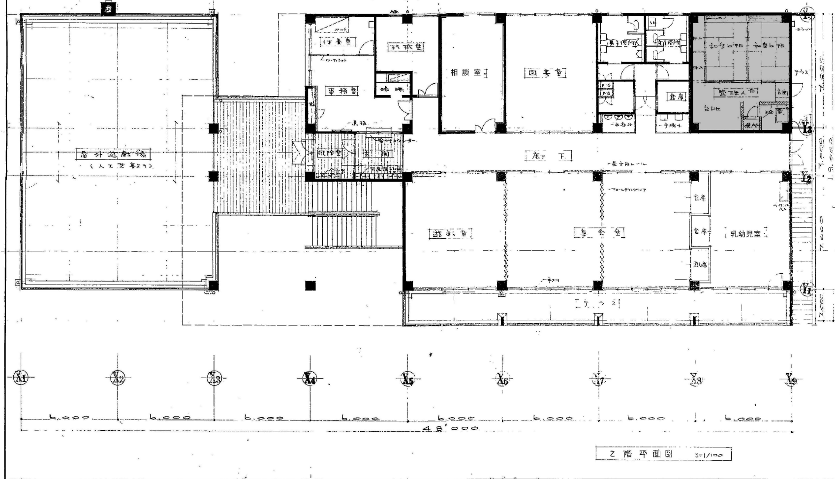
川口市立南平児童センター平面図
