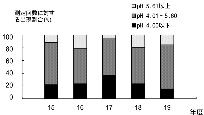
酸性雨出現割合の経年変化
