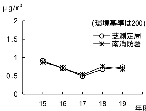
テトラクロロエチレン*年平均値の経年変化
