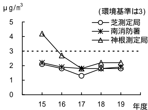
ベンゼン*年平均値の経年変化
