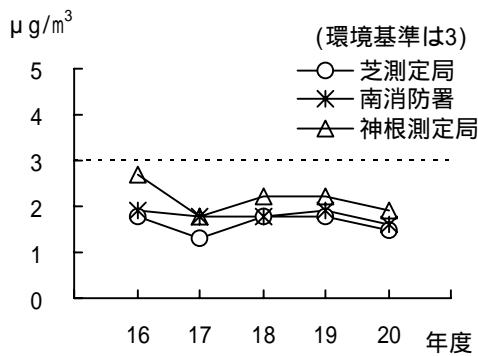
テトラクロロエチレン*年平均値の経年変化
