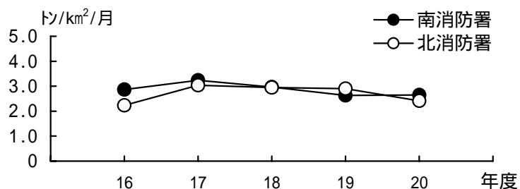
降下ばいじんの経年変化
