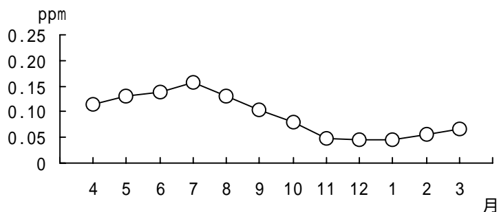
平成20年度 光化学オキシダント 月最高値の経月変化
