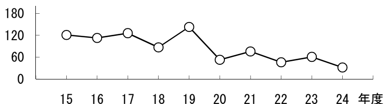
非メタン炭化水素濃度の午前6時から9時までの 3時間平均値が指針値（0.31ppmC）を超えた日数 日
