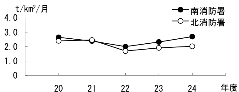
降下ばいじんの経年変化
