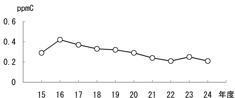
非メタン炭化水素午前6時から9時までの 3時間平均値の年平均値の経年変化
