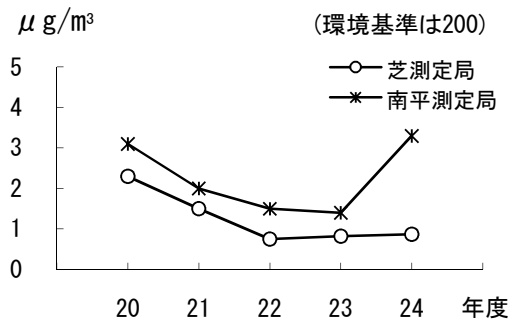
トリクロロエチレン年平均値の経年変化
