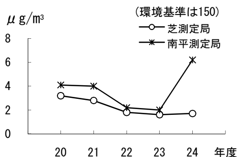
ジクロロメタン年平均値の経年変化
