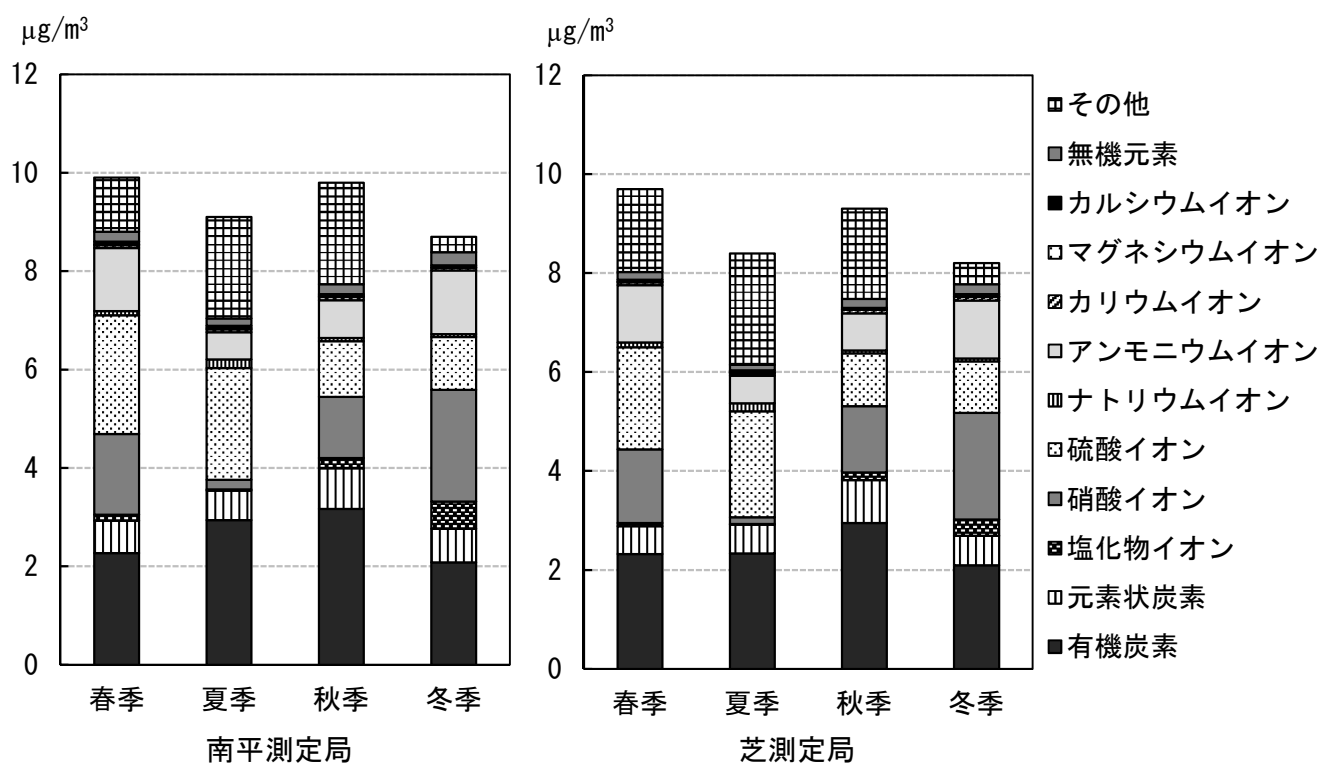
図 2.1.12 令和4年度 微小粒子状物質の成分濃度
