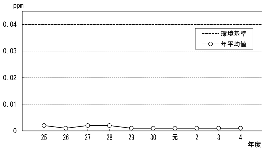
図 2.1.6 二酸化硫黄濃度の年平均値の経年変化
