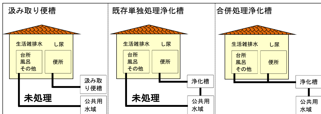
図 4.11 し尿・生活雑排水の処理方式
