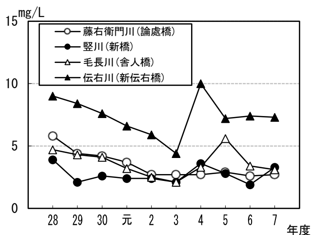
図 4.8 藤右衛門川等 4 河川 BOD75%値の経年変化
