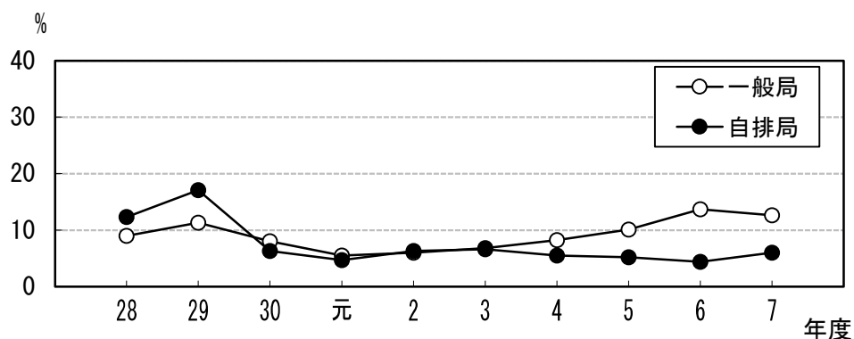
図 1.11 非メタン炭化水素濃度の午前 6 時から 9 時までの 3 時間平均値が指針値（0.31ppmC）を超えた日数の割合
