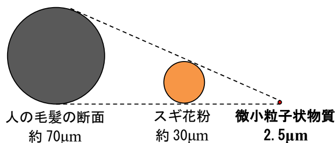
図 1.8 微小粒子状物質の大きさの比較
