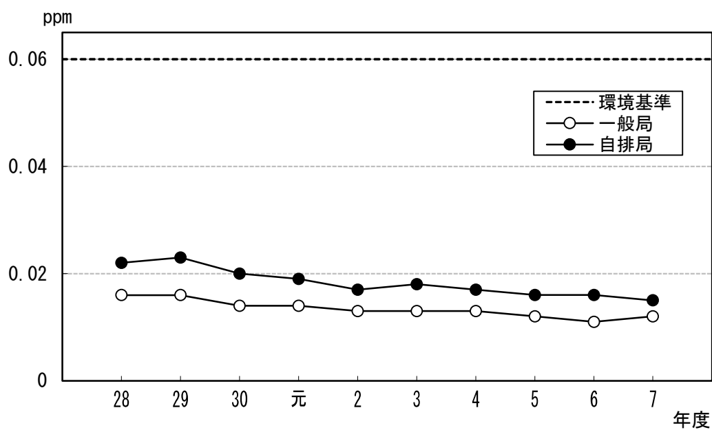
図 1.3 二酸化窒素濃度の年平均値の経年変化
