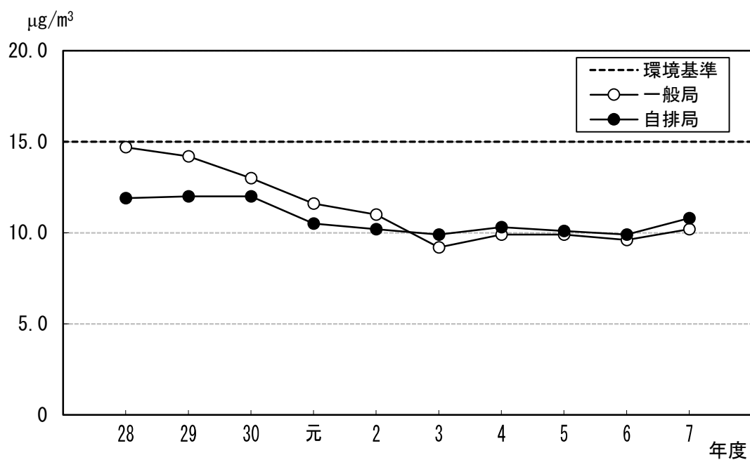
図 1.9 微小粒子状物質濃度の年平均値の経年変化
