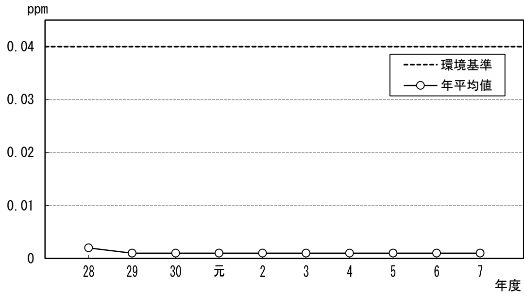
図 1.6 二酸化硫黄濃度の年平均値の経年変化
