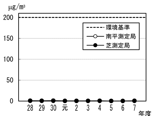
図 1.17 テトラクロロエチレン濃度の 年平均値の経年変化
