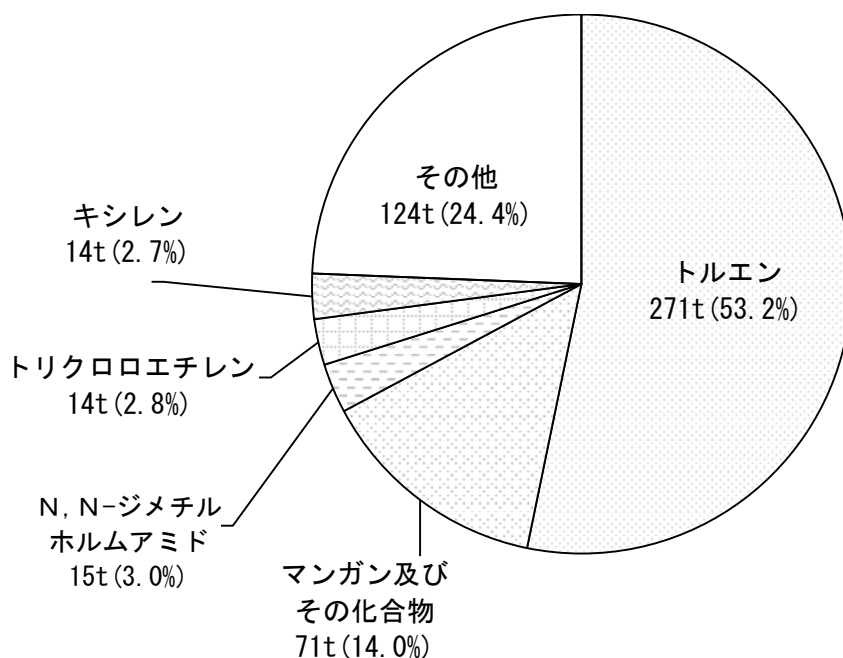
図 3.3 令和 6 年度 物質別排出量・移動量の合計と割合
