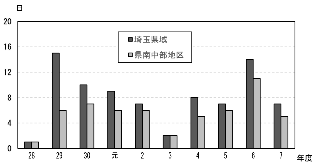
図 1.20 光化学スモッグ注意報発令日数の経年変化
