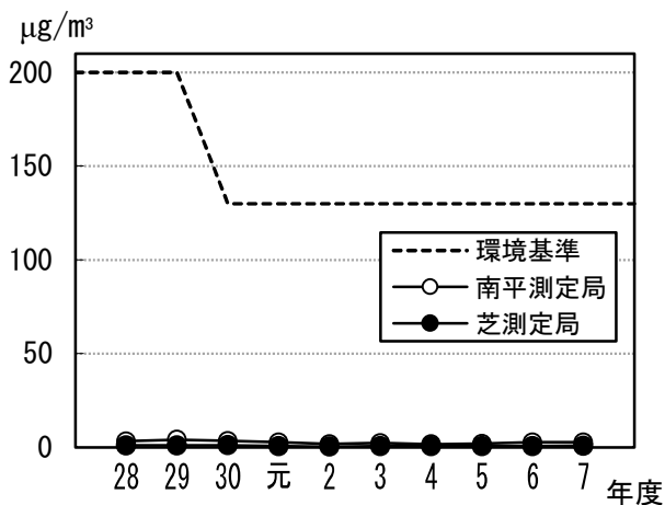
図 1.16 トリクロロエチレン濃度の 年平均値の経年変化
