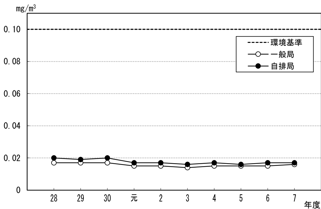
図 1.5 浮遊粒子状物質濃度の年平均値の経年変化
