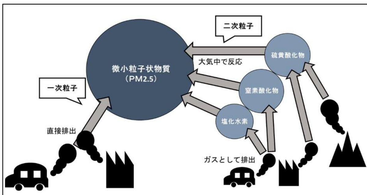
図 1.13 微小粒子状物質の主な生成メカニズム（模式図）
