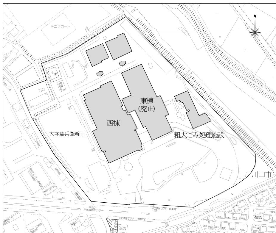
戸塚環境センター配置図
