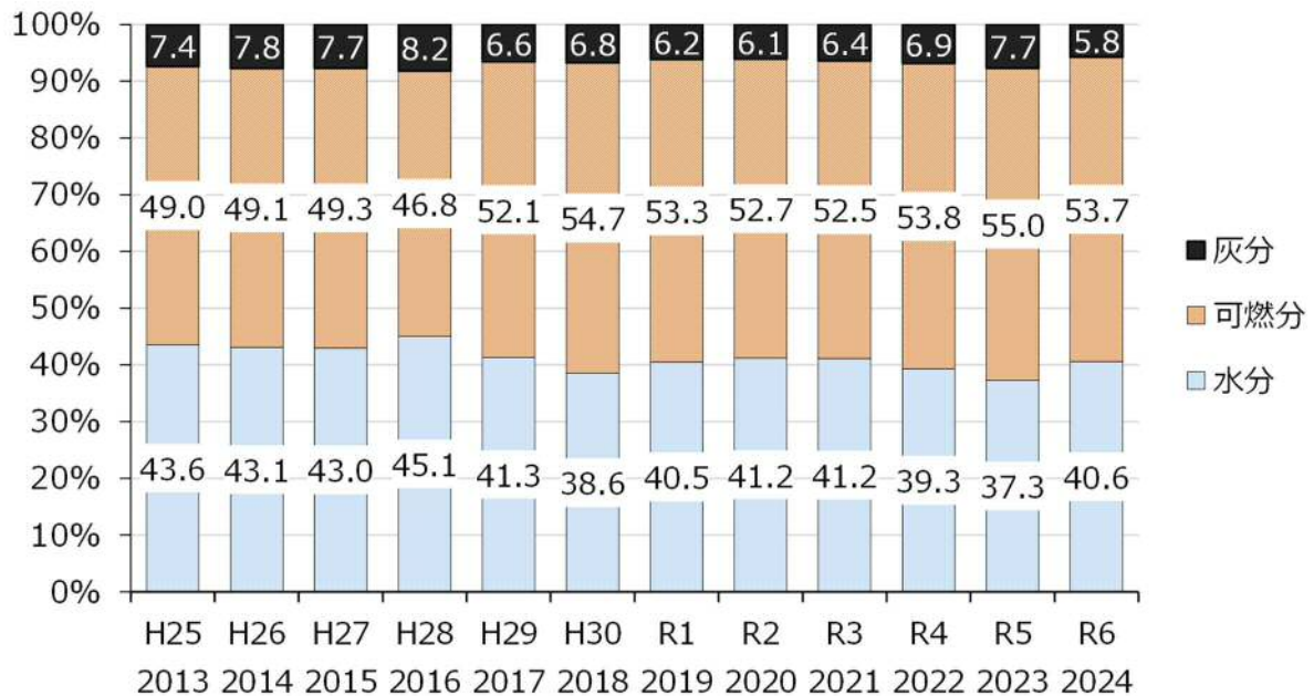
図表2-25 焼却対象ごみの3成分値（重量比）の推移（2センター平均）
