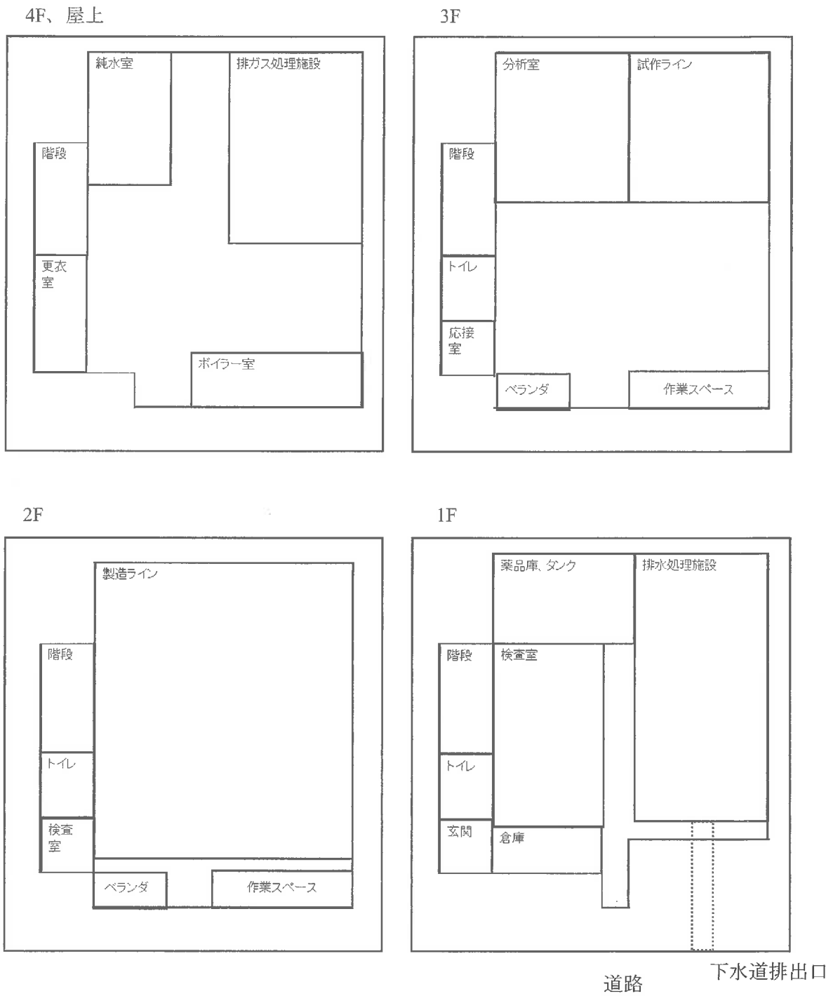
図3 工場配置図
