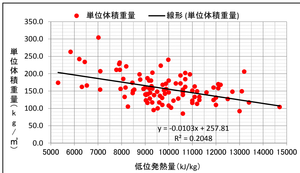
図2 低位発熱量と単位体積重量の関係
