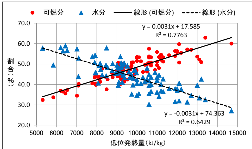
図1 低位発熱量と可燃分及び水分との関係
